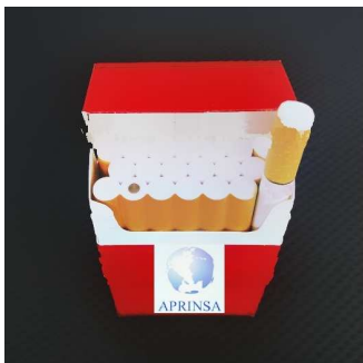
Bloqueador de Celulares Portatil Modelo 130A- 70x41x55mm Freq: CDMA 960 mhz, Gsm 1805-1990mhz, 3g:2110-2170mhz. Bloqueo 8 metros(señal >=-75dbm). Peso 70 Gramos. T.Operacion 90minutos
